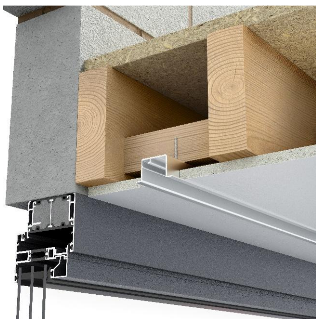
Profilé de rainure
