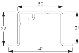
SG 11230 Nutprofil
