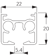
SG 11190 Profil
