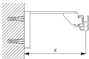
Smart Fix SG 11200 - SG 11205 et support SG 3603: Vis SG 10492 (M4x8) nécessaire.
