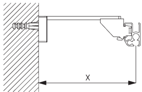
Square Smart Fix SG 11210 - SG 11215 et support SG 3603: Vis SG 10492 (M4x8) nécessaire.
