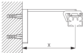
Smart Fix SG 11200 - SG 11205 et support SG 3826: Vis SG 10492 (M4x8) nécessaire.
