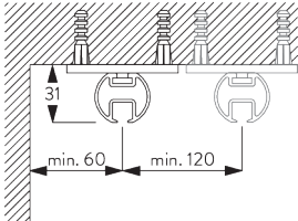
Träger SG 6124
