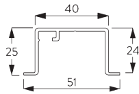
SG 10862 Nutprofil
