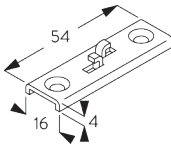
SG 6124 Träger
