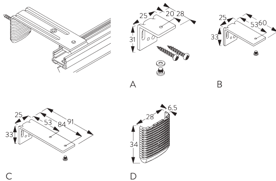
A: Supports-équerre 28 mm (M1) vis incluses B: Supports-équerre 60 mm (M2) vis incluses C: Supports-équerre 91 mm (M3) vis incluses D: Couverture pour supports-équerre
