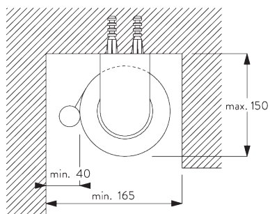
Rohr SG 4901 (ø 80 mm)
