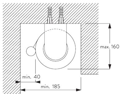
Rohr SG 4957 (ø 110 mm)
