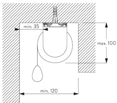
Montageprofil SG 11181 und Spanner SG 11180
