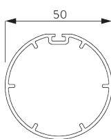
SG 2352 Profil
