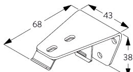
SG 2363 Träger 68 mm
